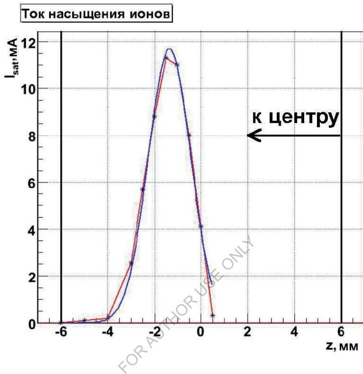
Рис. 4.7. Ток ионного насыщения в щели каспа. Точки, соединенные прямыми, – результат эксперимента, кривая – аппроксимация гауссовым профилем
