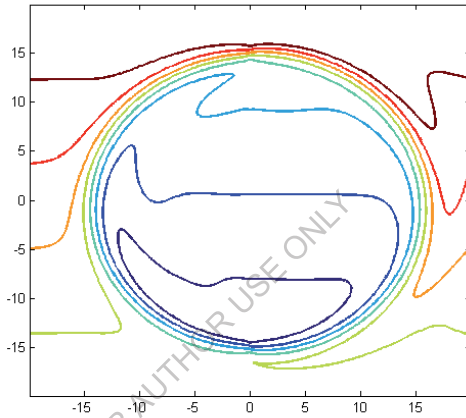
Рис. 3.32. Линии тока плазмы в сечении, перпендикулярном магнитному полю, при \Delta\varphi_w = T_e / e
