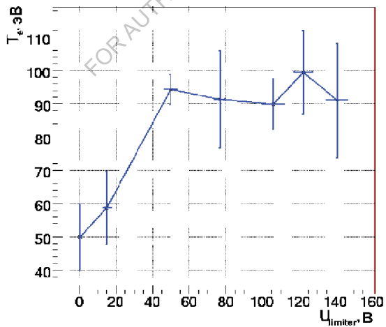
Рис. 3.22. Зависимость электронной температуры от напряжения на лимитере
