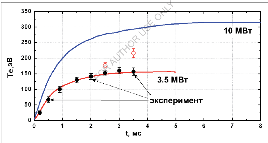
Рис. 3.26. Температура электронов плазмы по данным томсоновского рассеяния. За начало отсчета принят момент начала инжекции
