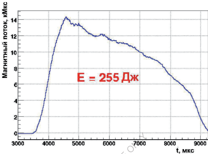
Рис. 4.2. Диамагнитный сигнал быстрых ионов при стабилизации расширителем
