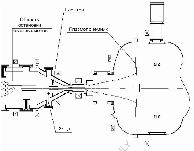
Рис. 2.3. Пробочный узел установки ГДП
