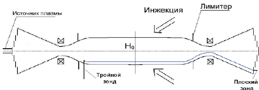
Рис. 3.28. Схема эксперимента по определению характера изучаемых колебаний
