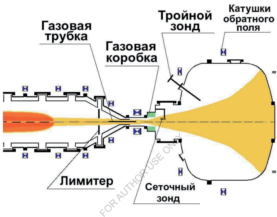
Рис. 4.1. Схема эксперимента с расширителем
