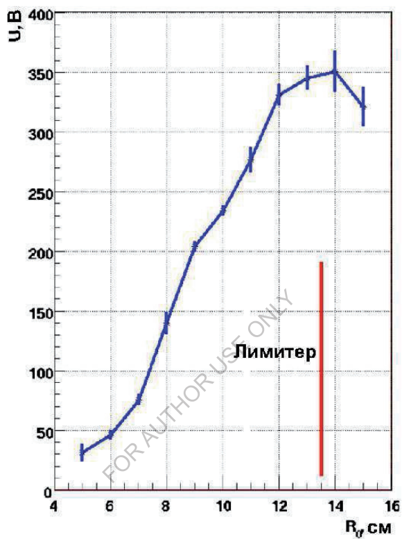
Рис. 3.36. Зависимость потенциала в плазме от радиуса при магнитном поле в центре установки B_0 = 2.5 кГс
