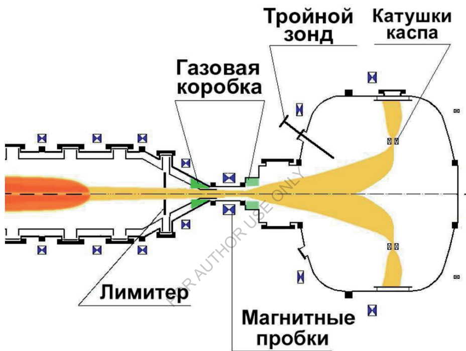
Рис. 4.3. Схема эксперимента с антипробкотроном
