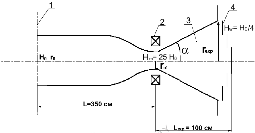
Рис. 1.1. Схематическое изображение половины центральной ячейки, пробки и расширителя установки ГДЛ: 1 – центральная плоскость, 2 – пробка, 3 – расширитель, 4 – приемник плазмы. (К вычислению коэффициентов уравнения (1.1))
