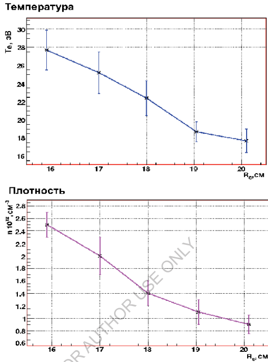
Рис. 2.8. Данные о плотности и электронной температуре окололимитерной плазмы
