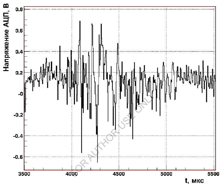
Рис. 2.5. Осциллограмма сигнала тока
