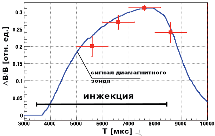
Рис. 3.27. Искажение магнитного поля по данным MSE-диагностики (точки) и диамагнитной петли (сплошная линия). Относительное давление плазмы
