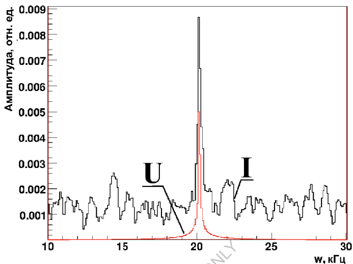
Рис. 2.7. Извлечение амплитуды сигнала тока при помощи Фурье-фильтра (амплитуда напряжения на рисунке уменьшена в 250 раз)
