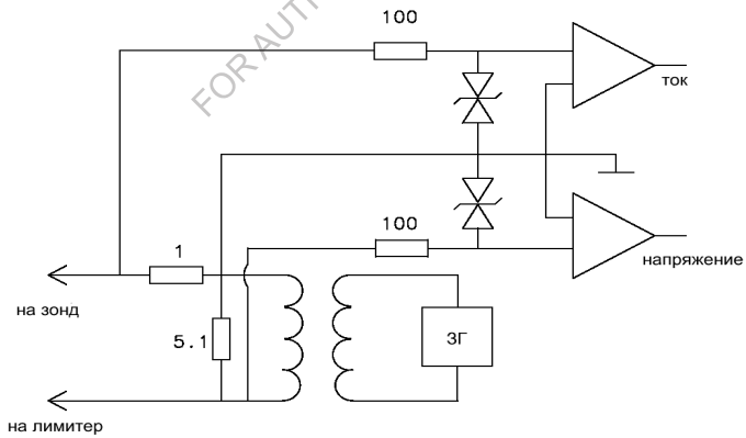
Рис. 2.4. Электрическая схема для измерения сопротивления дебаевского слоя лимитера
