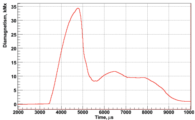
Рис. 3.19. Диамagnetный сигнал быстрых ионов при заземлении радиальных электродов. Сигнал получен при инъекции дейтериевых пучков
