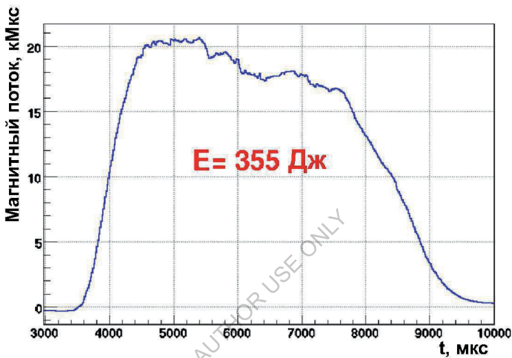
Рис. 4.5. Диамагнитный сигнал быстрых частиц в режиме стабилизации каспом при водородной инъекции
