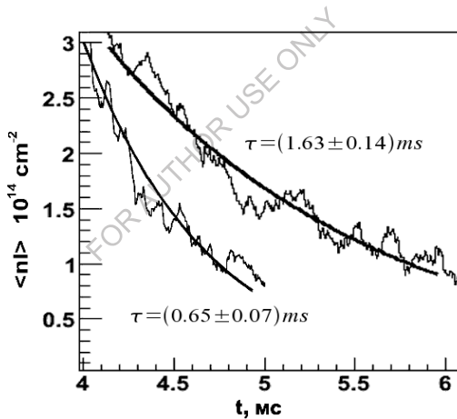
Рис. 3.10. Распад линейной плотности плазмы а – на лимитере и внешнем кольце плазмодриемника \approx 130 В, б – радиальные и торцевые электроды заземлены
