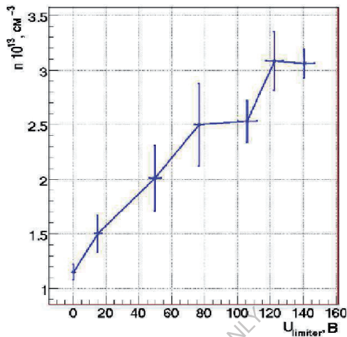
Рис. 3.23. Зависимость плотности электронов от напряжения на лимитере
