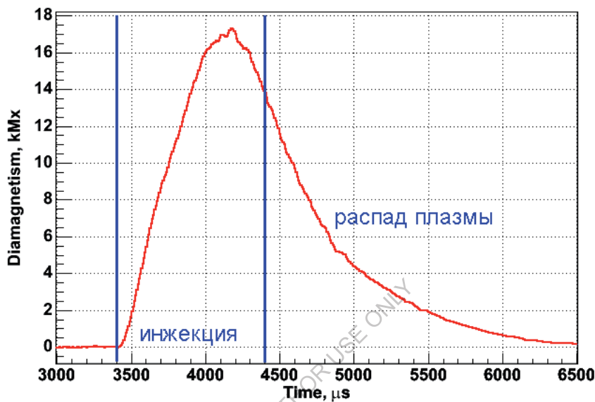
Рис. 3.4. Диамагнитный сигнал быстрых частиц
