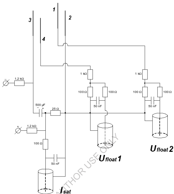
Рис. 3.14. Электрическая схема комбинированного зонда
