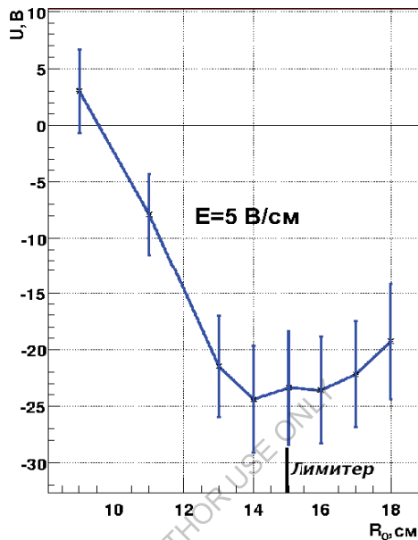
Рис. 3.3. Профиль потенциала плазмы при отрицательном смещении на лимитере (-25 В)
