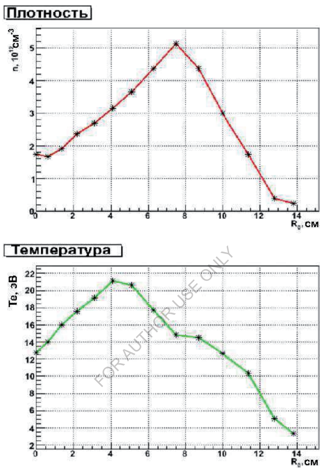
Рис. 4.4. Температура и плотность плазмы в расширительном баке при стабилизации каспом
