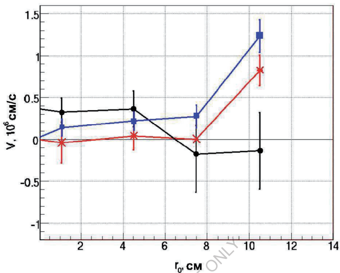
Рис. 3.34. Радиальные профили азимутальной скорости вращения плазмы.
