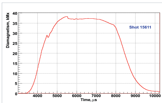
Рис. 3.17. Диамагнитный сигнал быстрых ионов при подаче на лимитер потенциала \approx 180\text{В} . Сигнал получен при инъекции дейтериевых пучков
