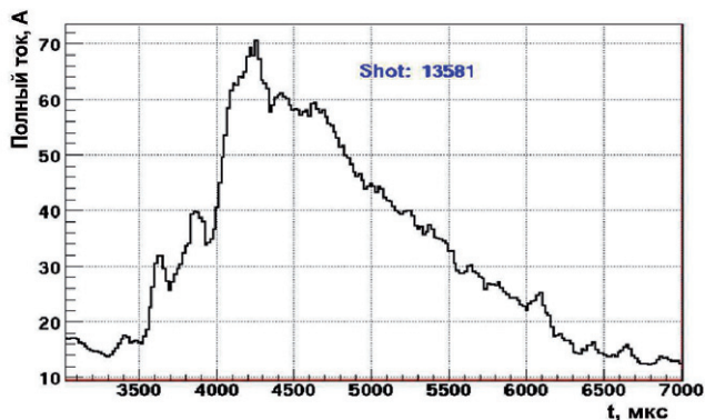
Рис. 3.33. Полный ток, текущий на кольцо плазмоприемника, проецирующееся на область перепада радиального потенциала в центральной ячейке
